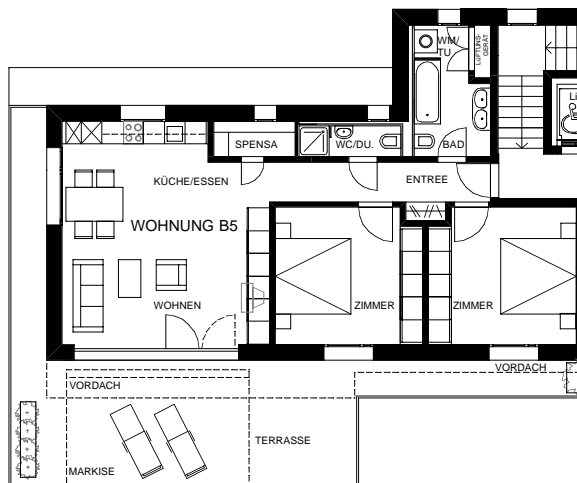
Dachgeschoss
