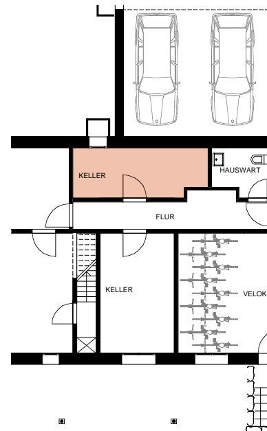
Untergeschoss
