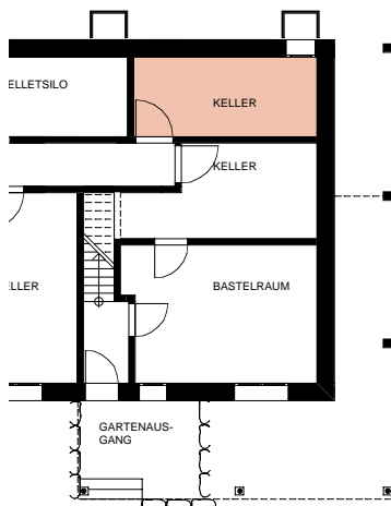
Untergeschoss
